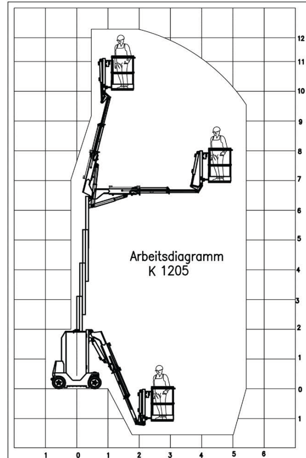
Arbeitsdiagramm (Arbeitsbereich)
